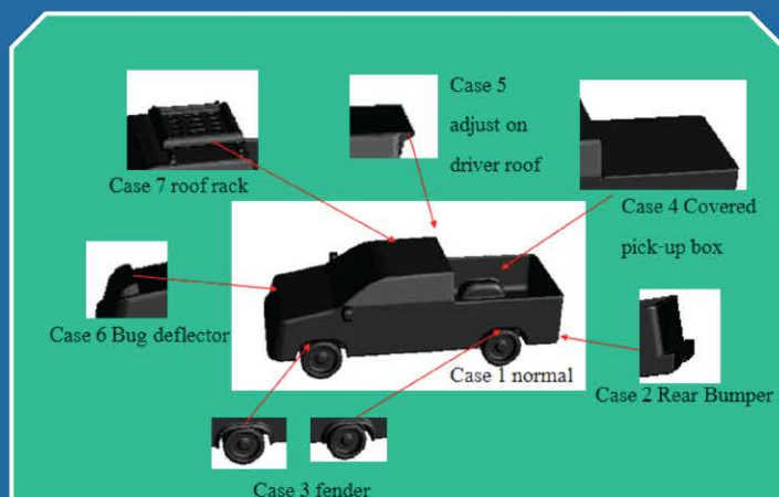
รูปที่ 4 ตำแหน่งและกรณีที่ติดอุปกรณ์เสริมโดยวิธีจำลอง CFD
